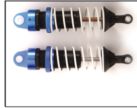
6014 Stoßdämpfer (Aluteile) Shock absorber unit (alu parts)
